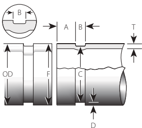
Roll Groove
