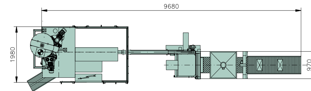
Dettaglio magazzino sacchi Bag warehouse detail Détail de l'entrepôt de sacs
