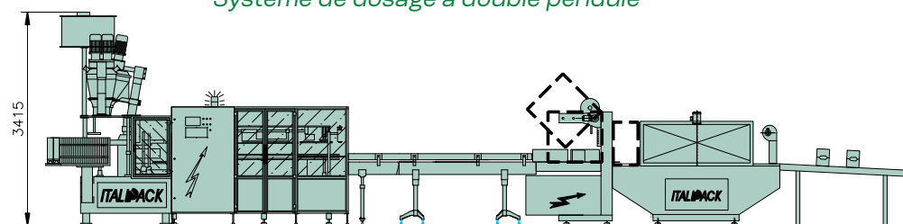
Sistema a due dosatori pendolari doppi Double pendulum dosing system Système de dosage à double pendule
