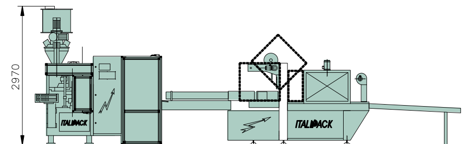
Sistema Aspirazione polveri Dust vacuum system Système d'aspiration des poussières
