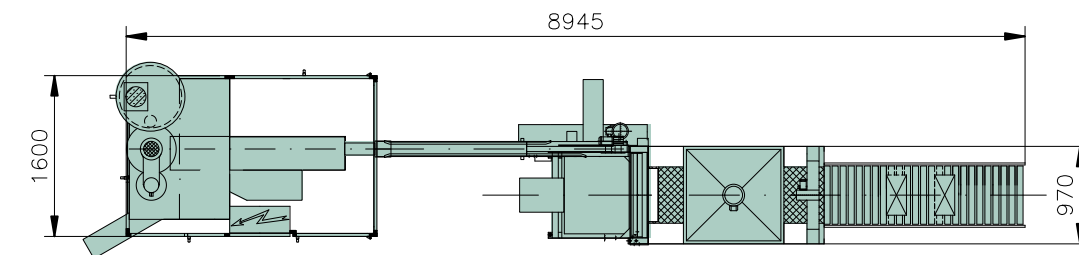
Dosatore volumetrico singolo per granulari Single volumetric dosing unit for granulars Unité de dosage volumétrique unique pour les granulés
