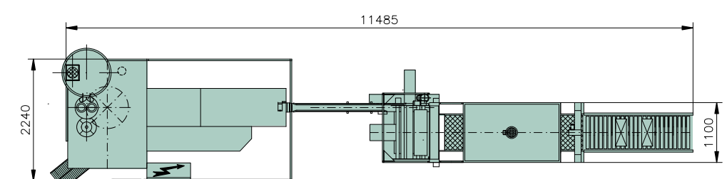
Dosatore volumetrico doppio per granulari Double volumetric dosing unit for granulars Unité de dosage volumétrique double pour granulés
