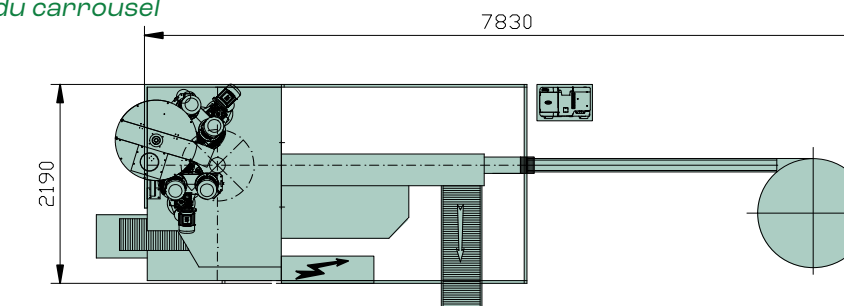
Dettaglio carosello Carousel detail Détails du carrousel
