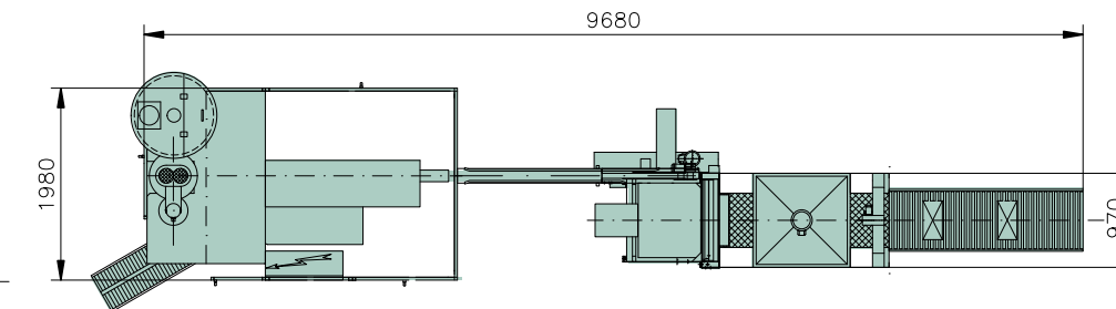
Dosatore volumetrico doppio per granulari Double volumetric dosing unit for granulars Unité de dosage volumétrique double pour granulés
