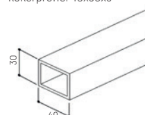
Art. nr. 12741 kokerprofiel 40x30x3
