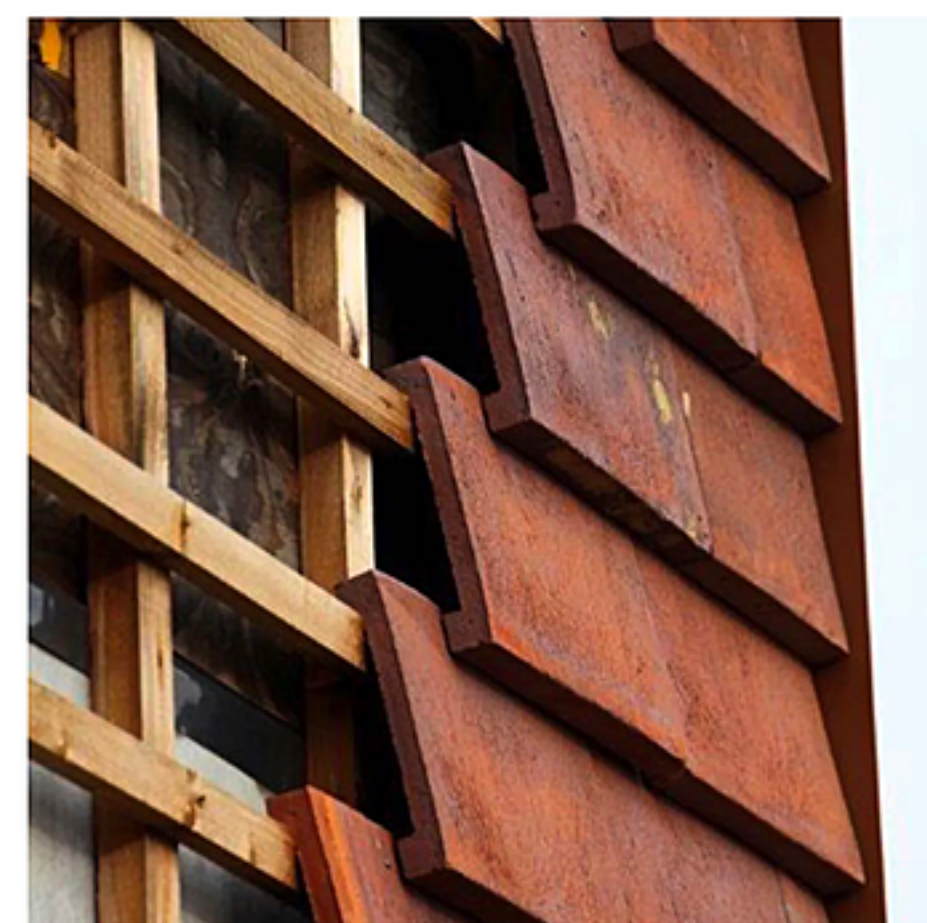
Unterkonstruktion und Eckfügung
