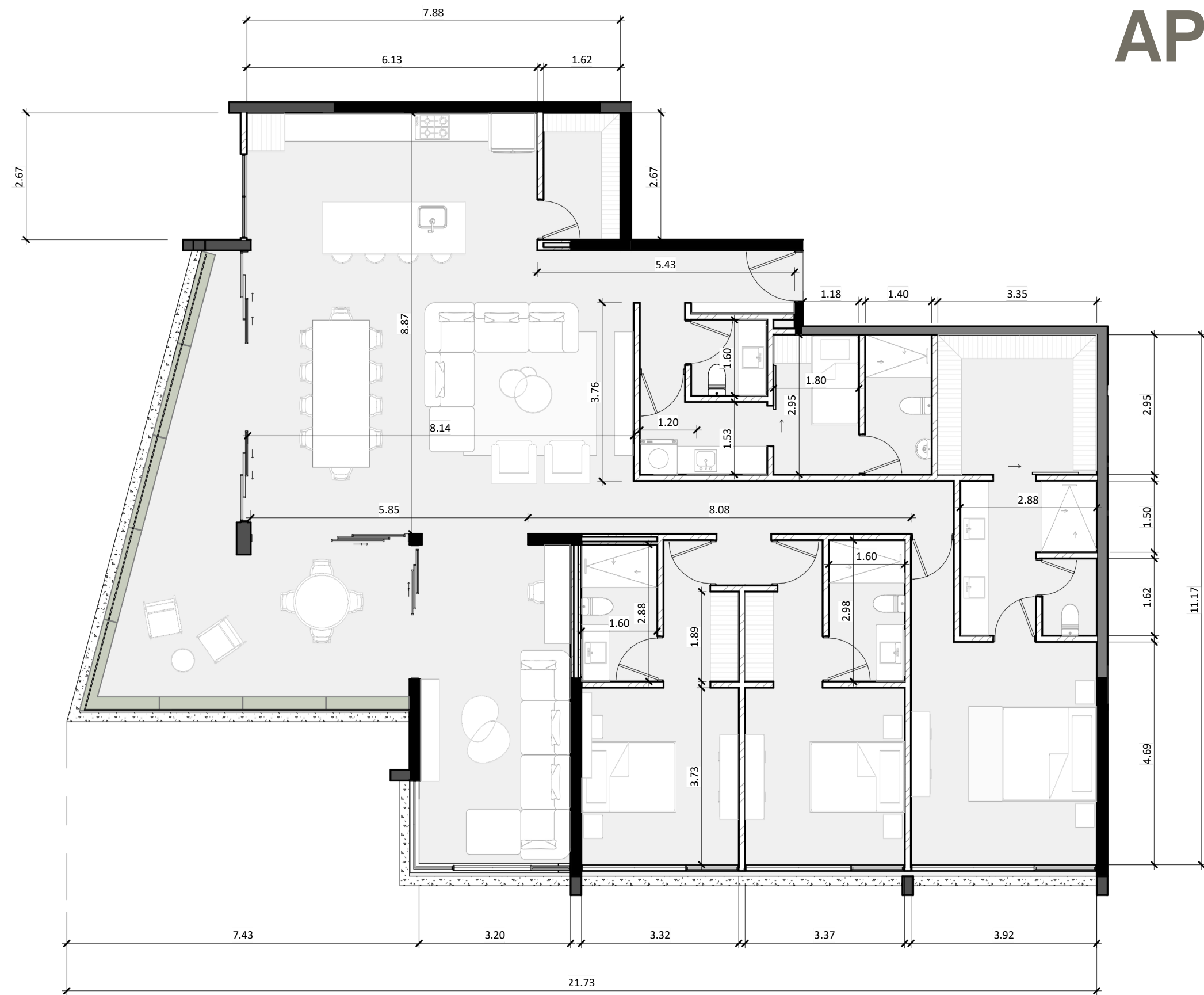
PLANTA DE DISTRIBUCIÓN
