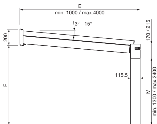
GP3100 Seitenansicht
