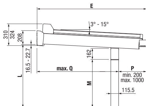
GP4200 Seitenansicht
