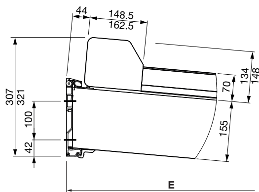
GP3100 Wandanschluss
