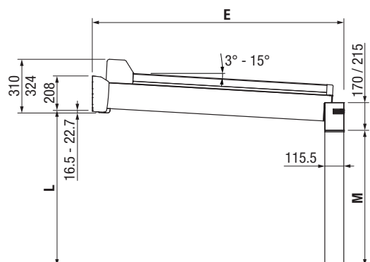
GP4100 Seitenansicht
