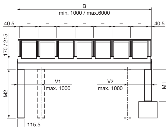
GP3100 Frontansicht
