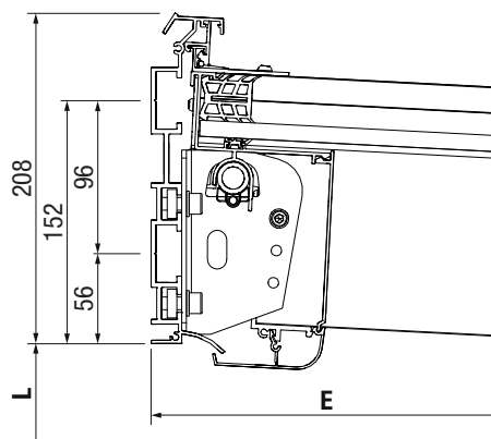
GP4100 Wandanschluss
