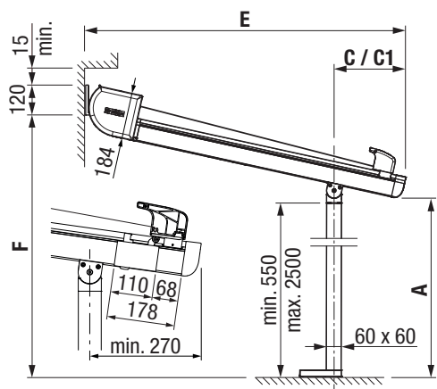
P3600 Wandmontage mit Fussplatte
