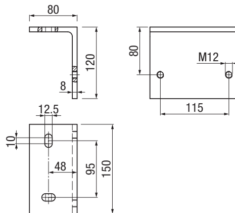
P3600 P333 Deckenwinkel
