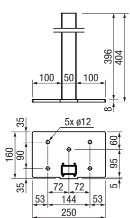
P3600 P363 Fussplatte
