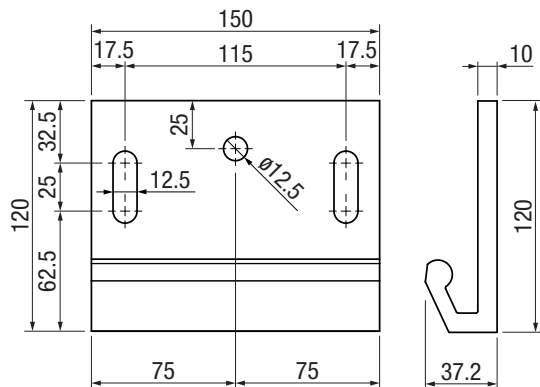
P3600 Konsole Standard
