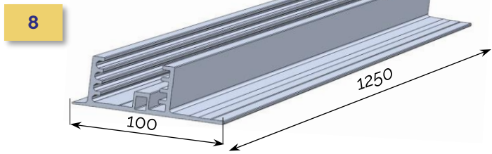
EMBASE PAYSAGE 1250 mm
