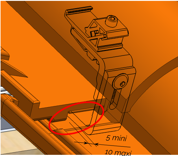
Vue en coupe sur tuile plate.
