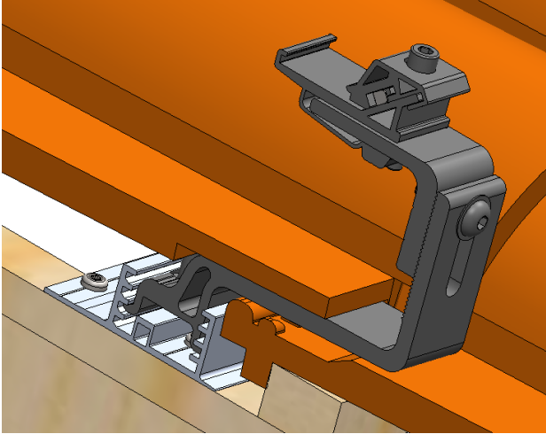
Vue en coupe sur tuile plate.
