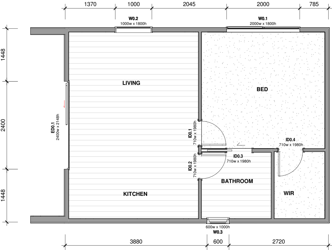
W & D SET OUT PLAN 1 : 50
