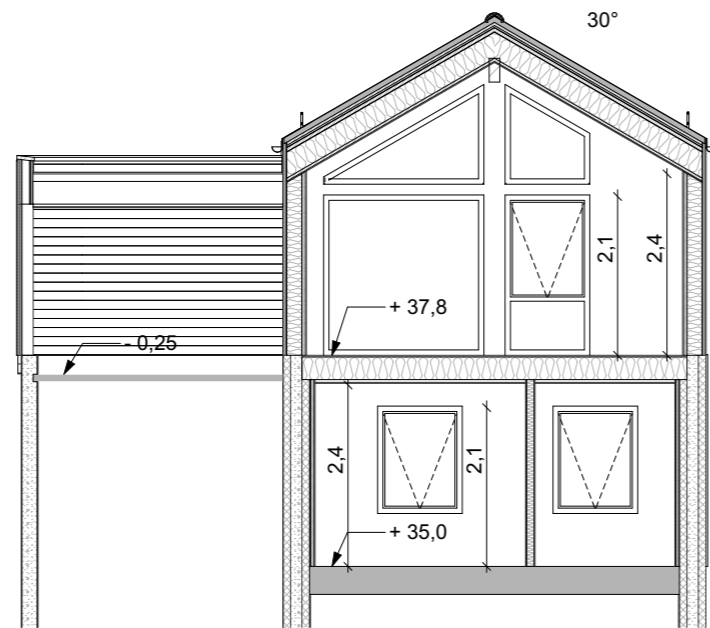
Snitt A
