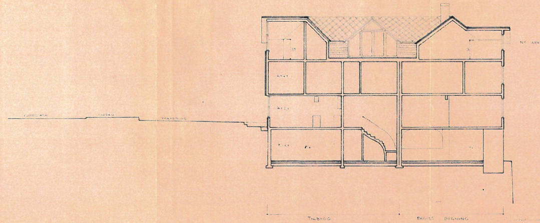
SNITT 0-0 FRA FJØRA MOT SJØEN
