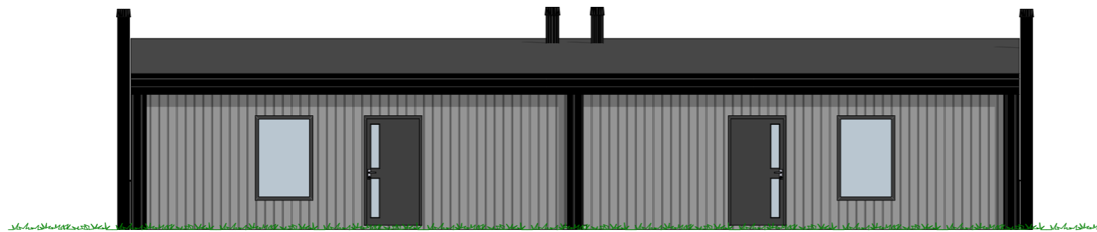
1:100 Fasade Vest
