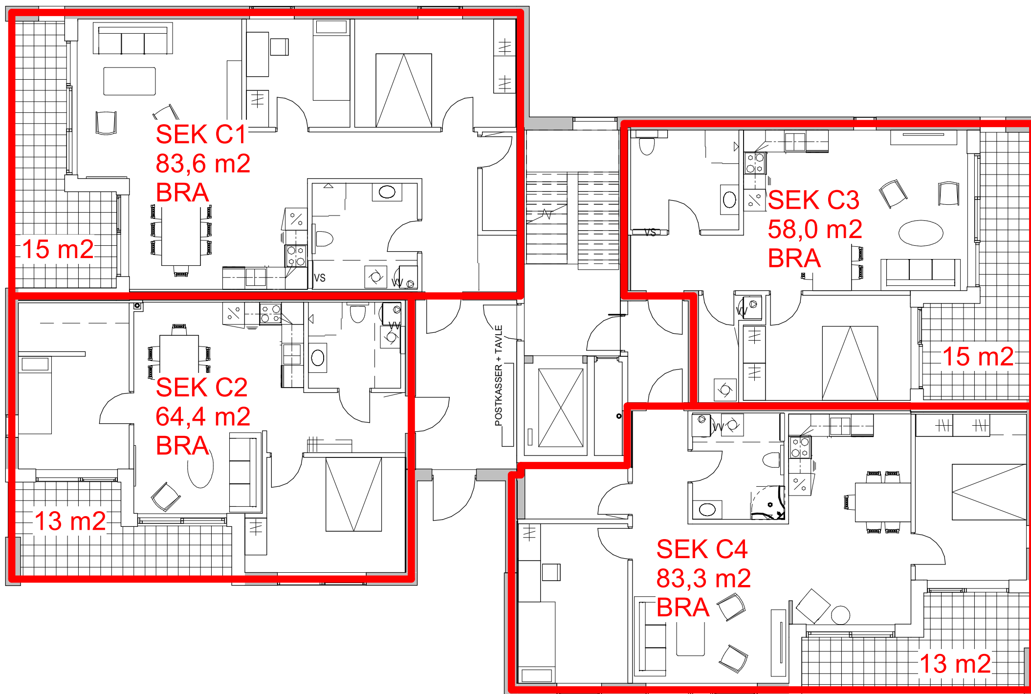
BYGG C PLAN 1 1:100
