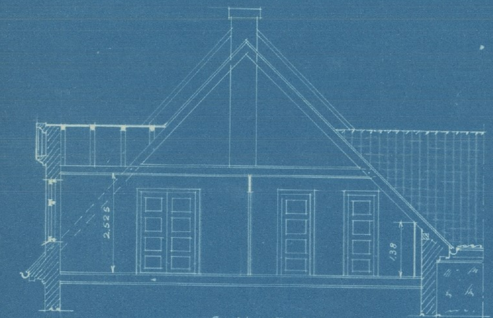
Snit - A-A
