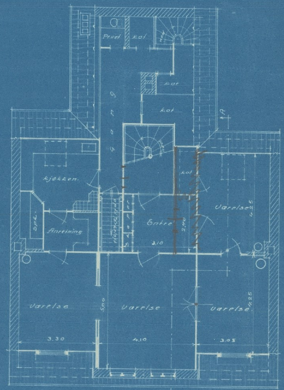
Plan av Lofteloge
