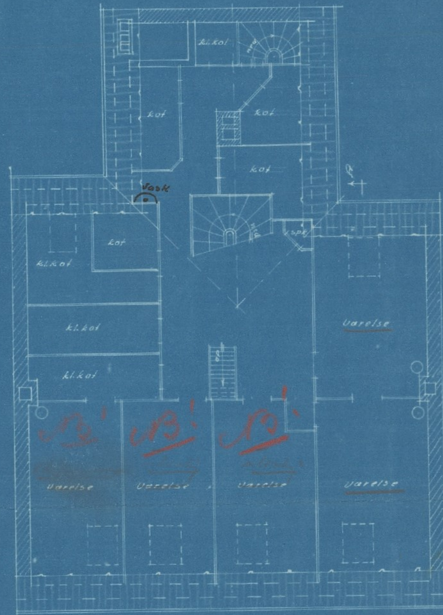
Plan av Loftetage
