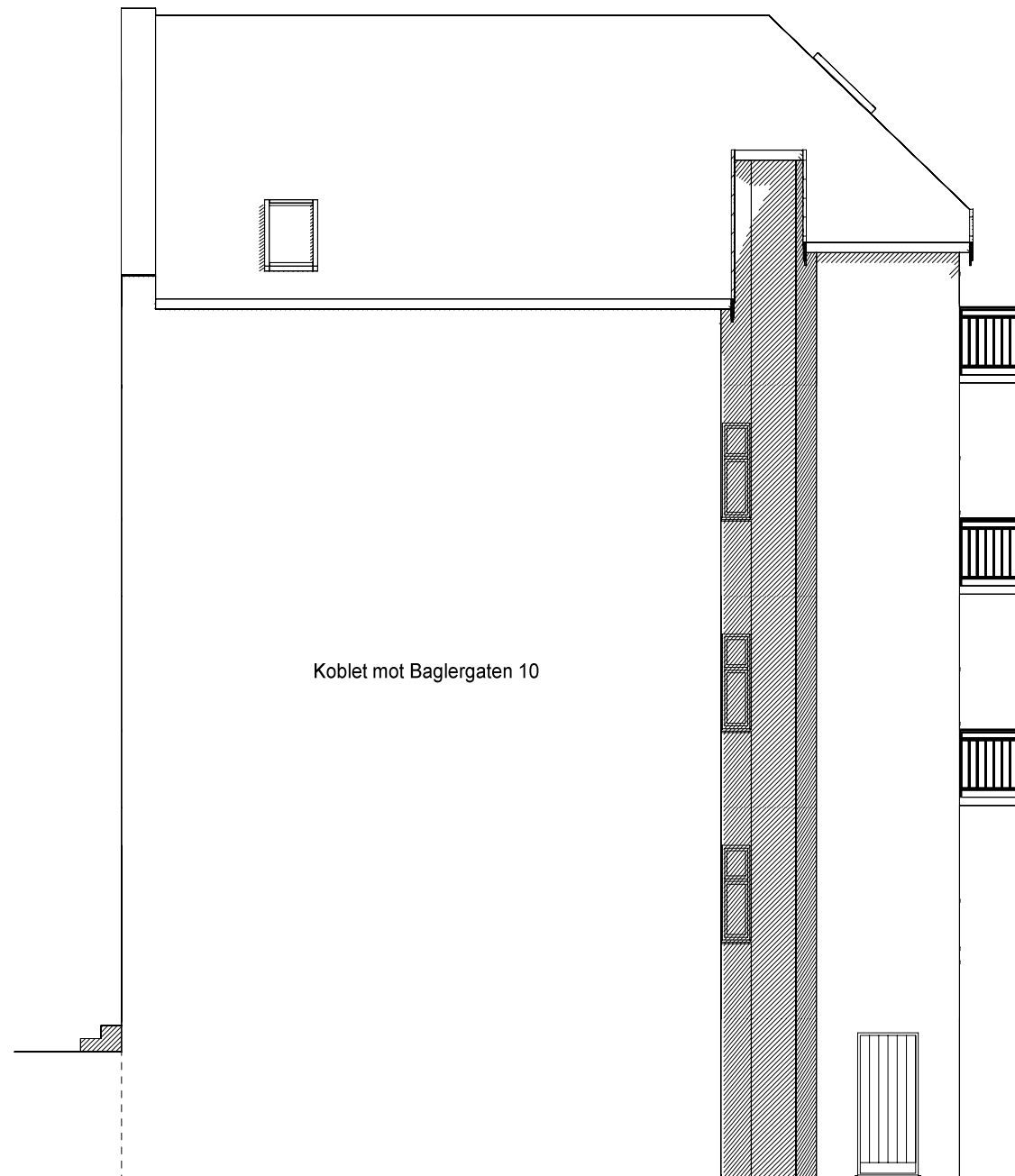
FASADE MOT NORD-ØST Ny situasjon
