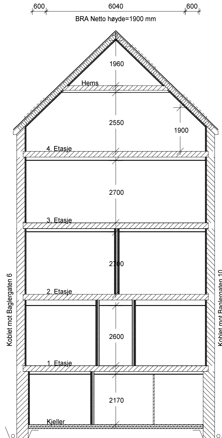
SNITT A-A Ny situasjon
