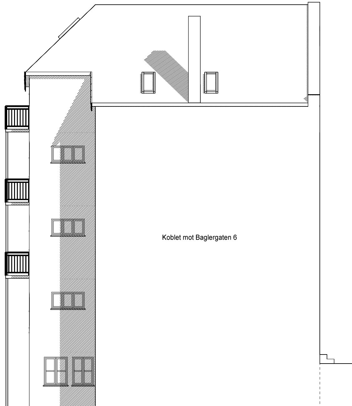
FASADE MOT SØR-VEST Ny situasjon
