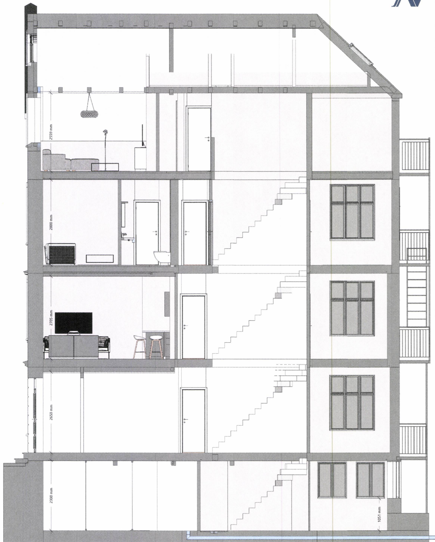
Baglergaten 8 - snitt A
