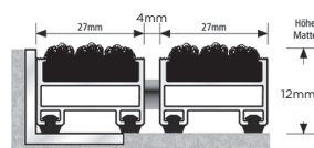
PROFIL
