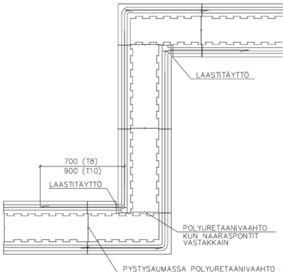
Kuva 4. Nurkan rauditus.
