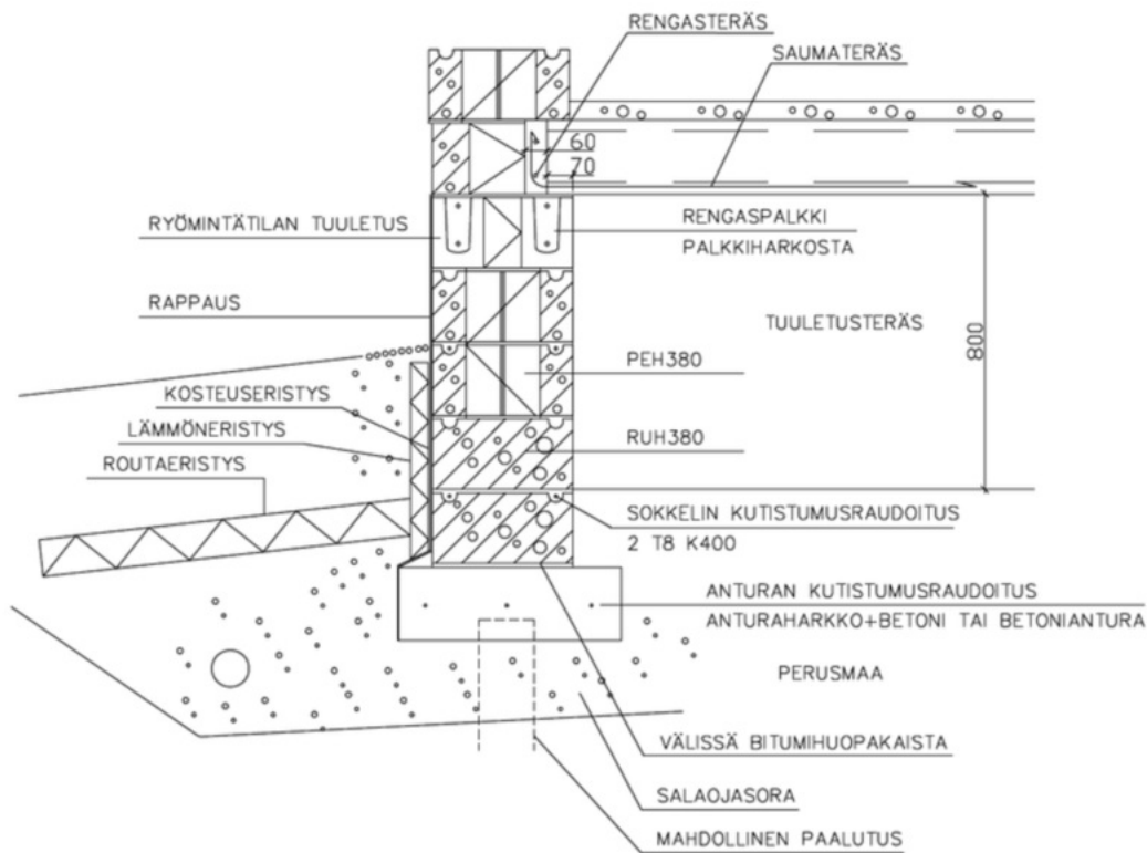
Kuva 6. Ryömintätillainen perustus.
