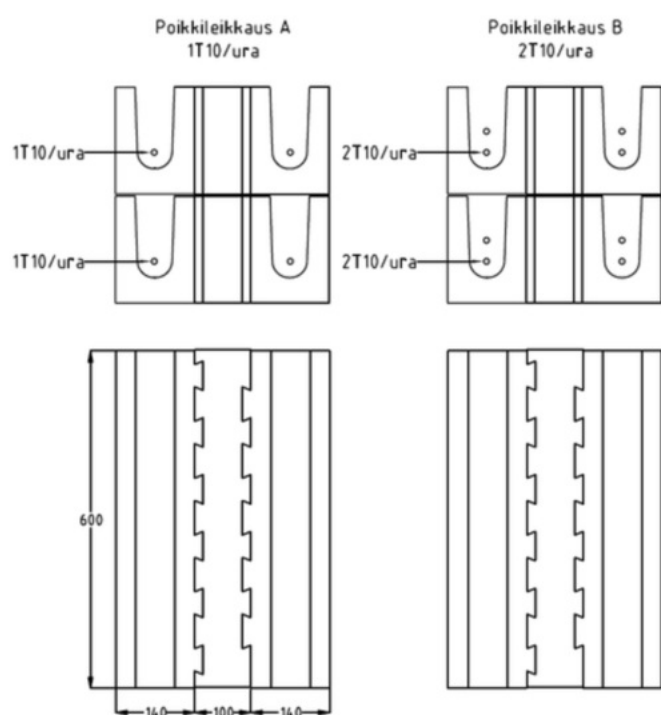
Kuva 8. Palkkiharkon raudoitus.
