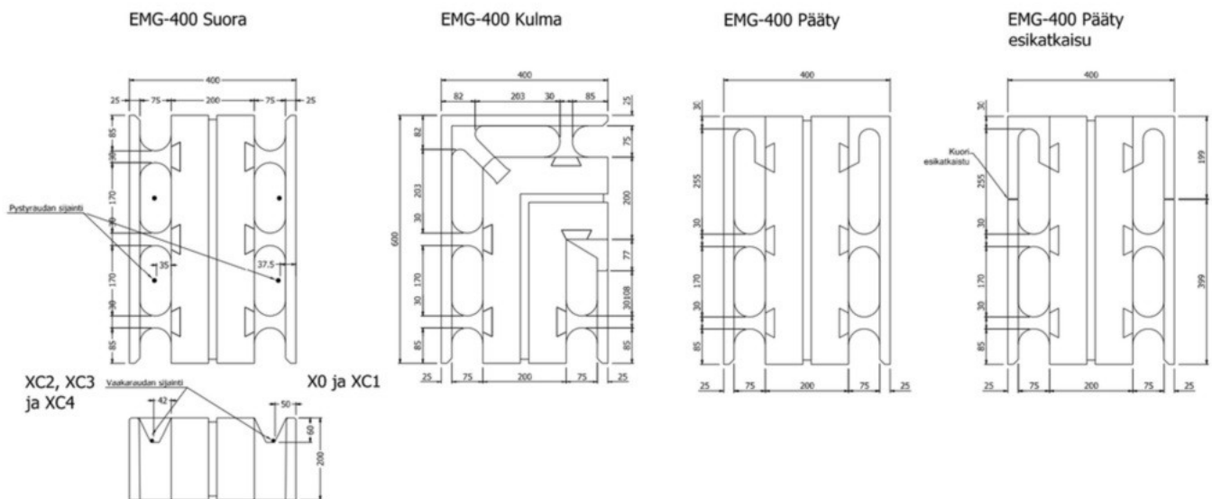
Kuva 1. Mittakuvat.
