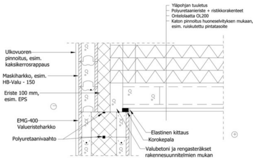
Kuva 14. Ontelolaatan liitos.
