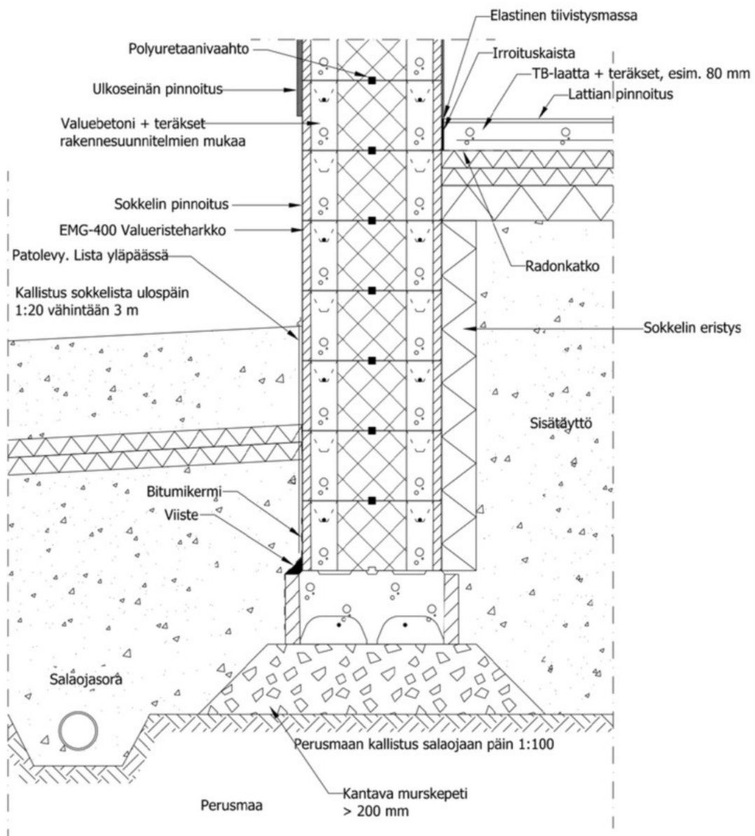
Liite 2. Perustusleikkaus.
