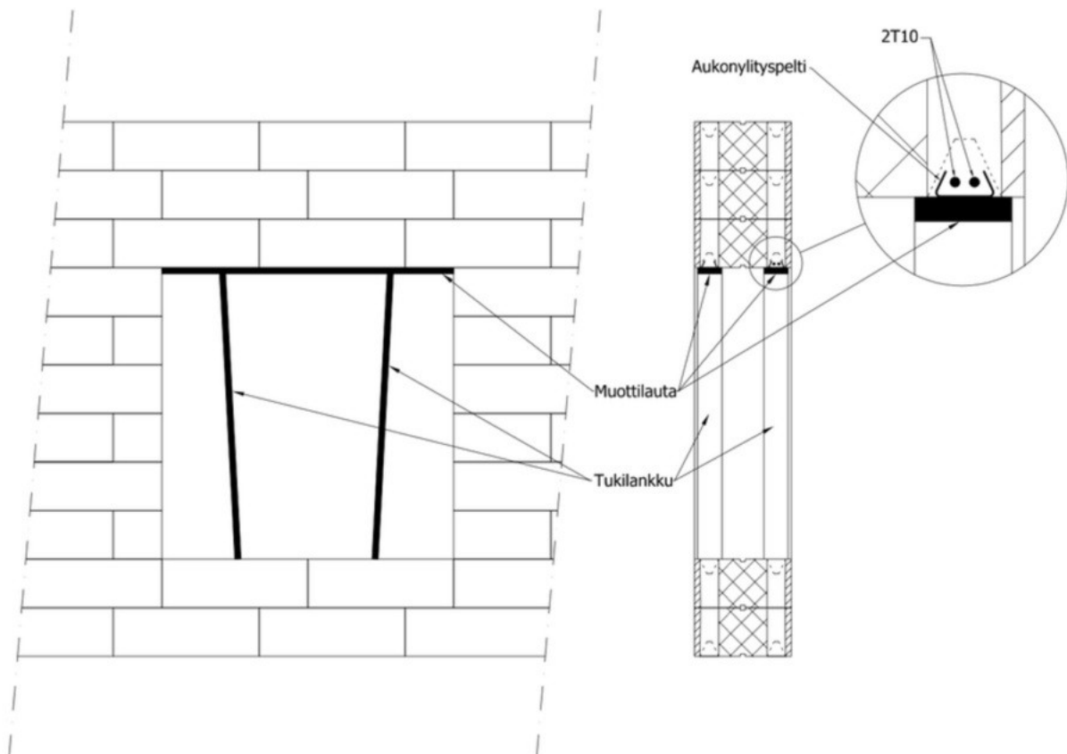
Kuva 4. Aukon ylitys.
