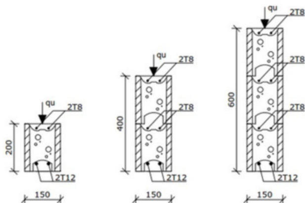
Kuva 8. Leikkausraudoittamaton palkki.
