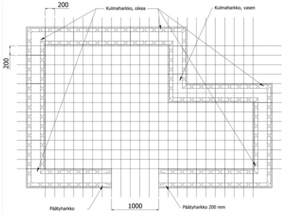
Kuva 2. Moduulimitoitus.
