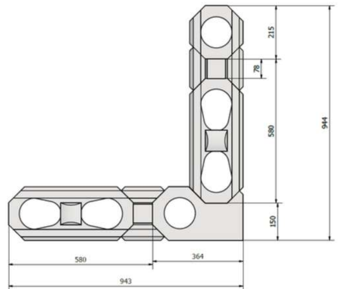
Kuva 2. Vallikivi L-kulma ilman kivien sahaamista -kaava.
