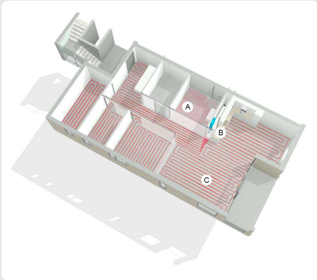
Figur 1: Leggemønster for leilighet
