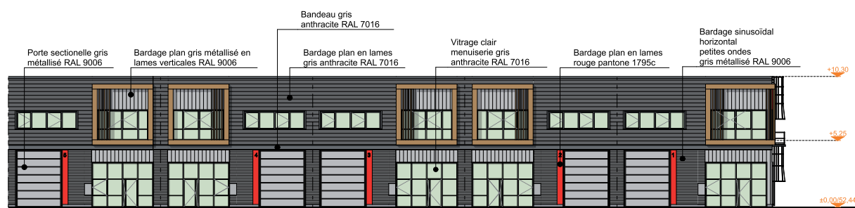
Façade Est
