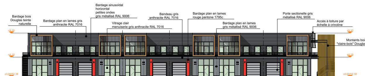
Façade Ouest
