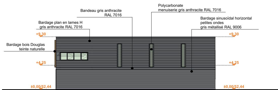
Façade Sud
