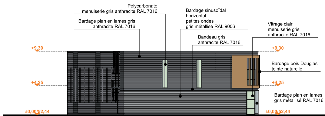
Façade Nord
