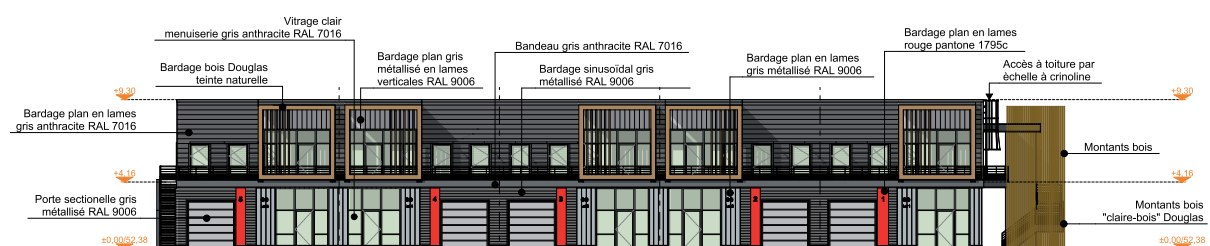
Façade Sud
