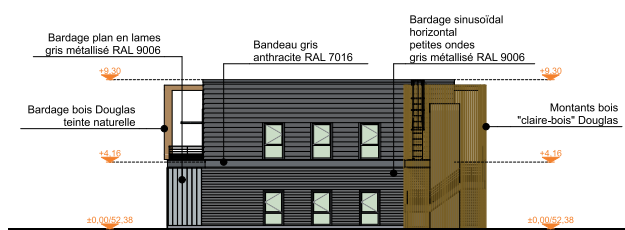
Façade Sud
