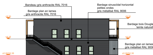
Façade Ouest
