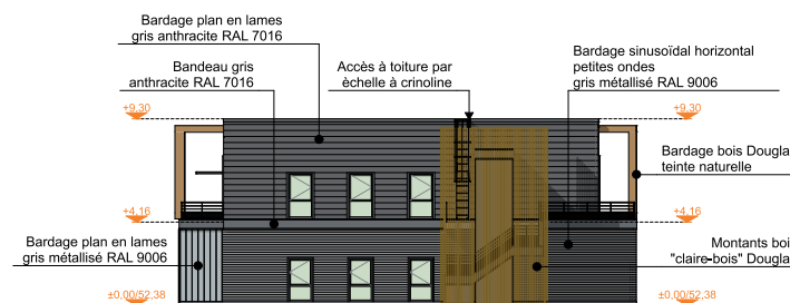
Façade Est
