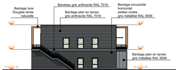
Façade Nord
