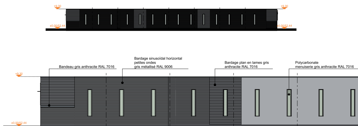
Façade Est
