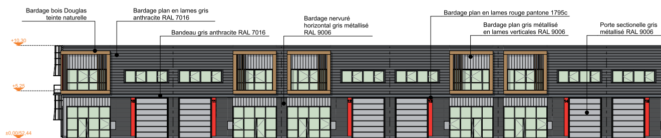
Façade Ouest
