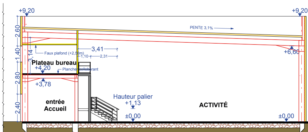
COUPE B3
