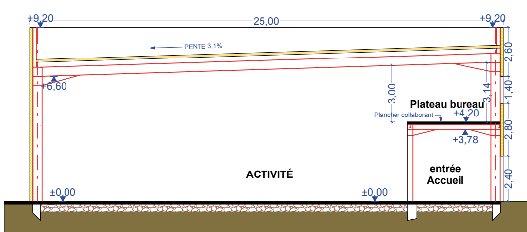
Coupe de principe AA (sur entrée activité bâtiment A)
