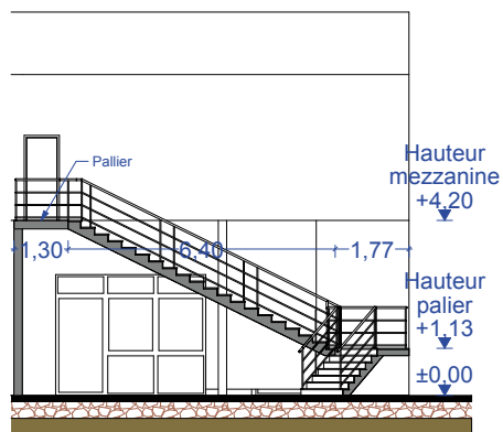
COUPE B2
