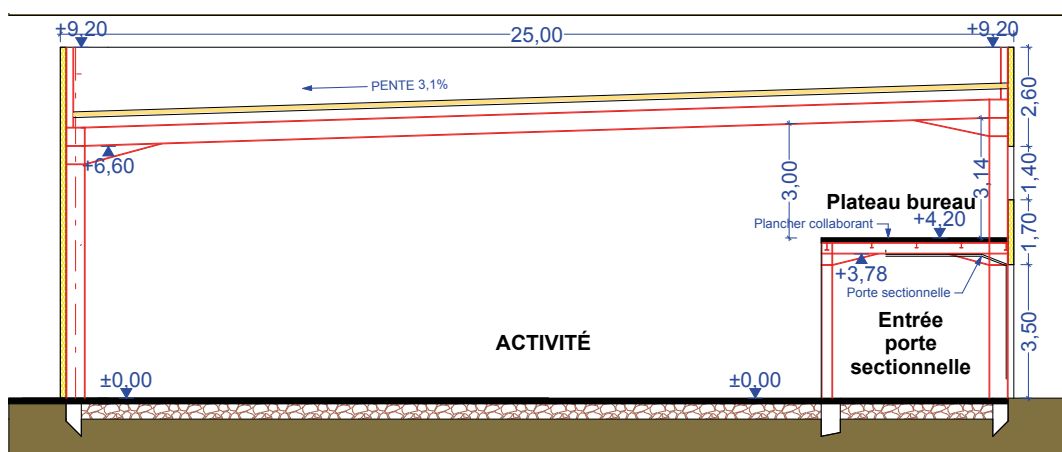
Coupe de principe AA (sur accueil bâtiment A)
