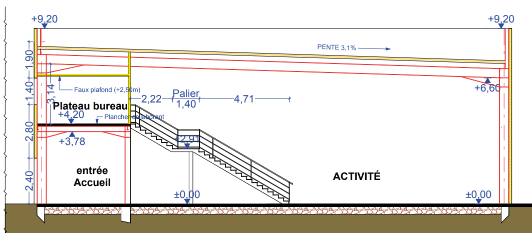
Coupe de principe BB (sur entrée activité bâtiment B)
