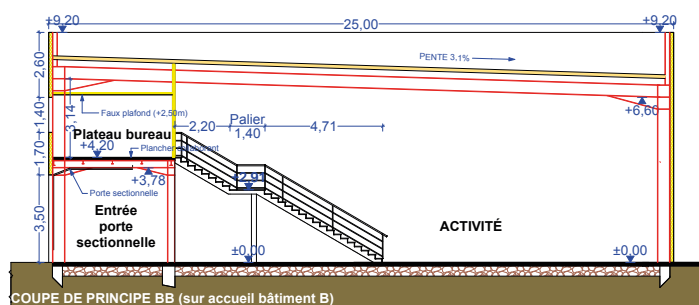
COUPE DE PRINCIPAL
