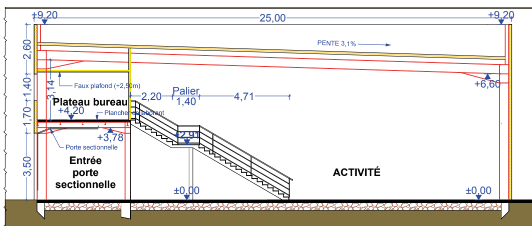
Coupe de principe BB (sur accueil bâtiment B)
