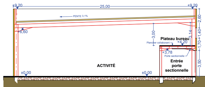
COUPE DE PRINCIPE
