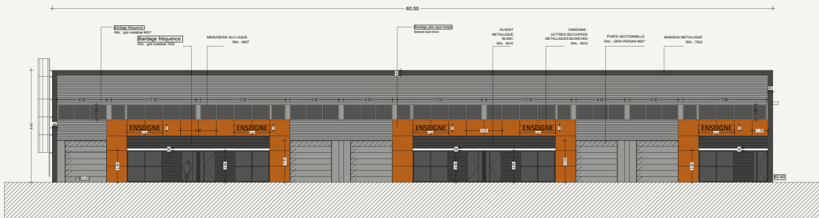
FACADE OUEST BAT 4 1/250 - PC5
