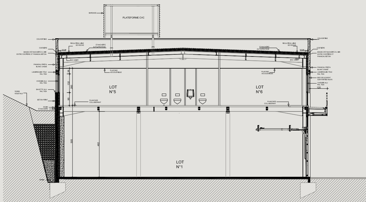
COUPE BB
