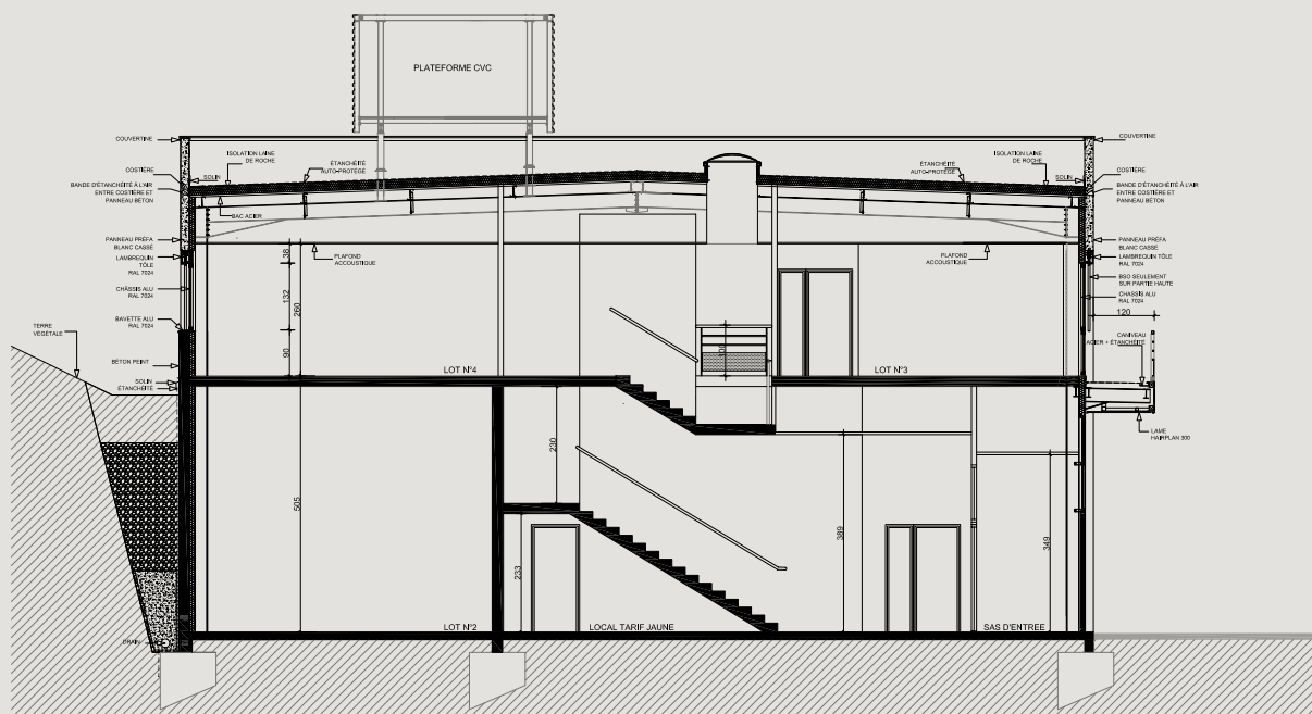
COUPE AA
