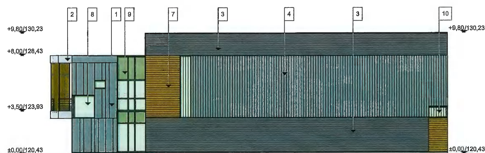
FACADE NORD-EST
