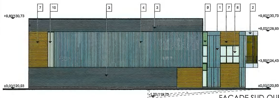
FACADE SUD-OUEST
