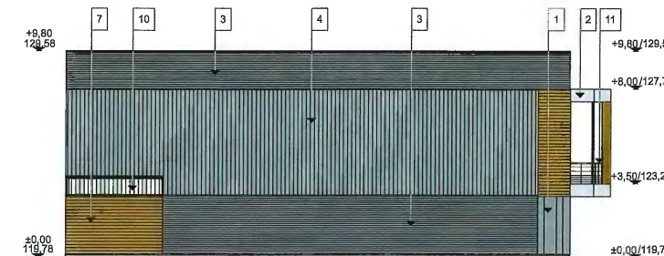
FACADE SUD-EST
