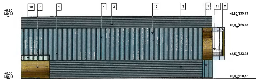
FACADE NORD-OUEST
