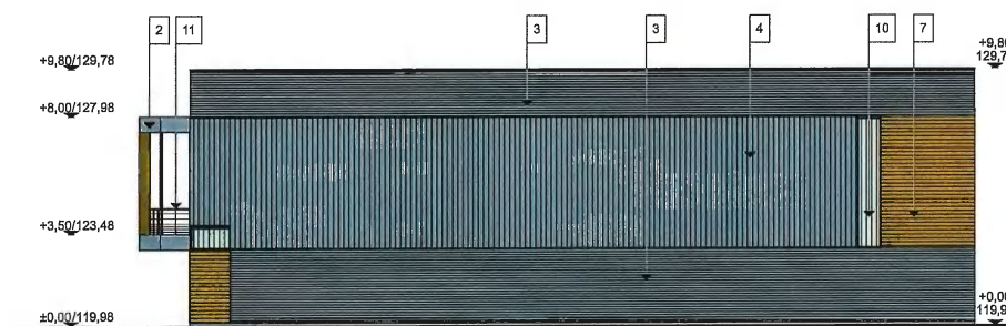
FACADE SUD-EST
