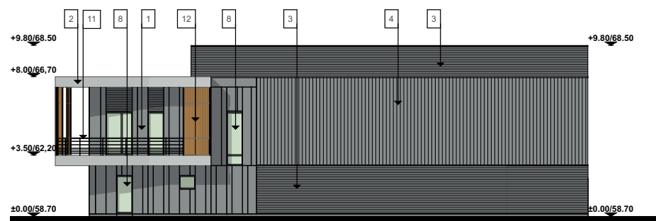
FACADE NORD
