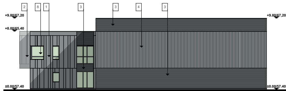
FACADE EST
