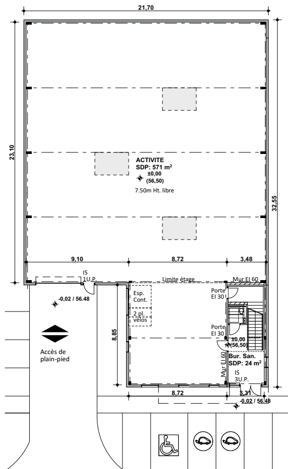
PLAN DU REZ-DE-CHAUSSEE
