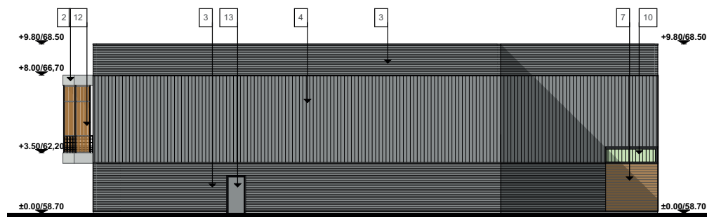
FACADE OUEST
