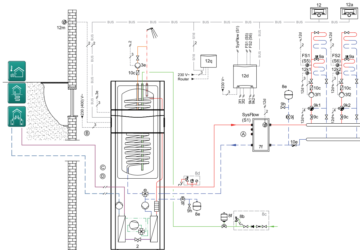
Installatievoorbeeld 2: flexoCOMPACT VWF ..8/4 met 2 verwarmingscircuits en een buffervat als hydraulische scheiding
