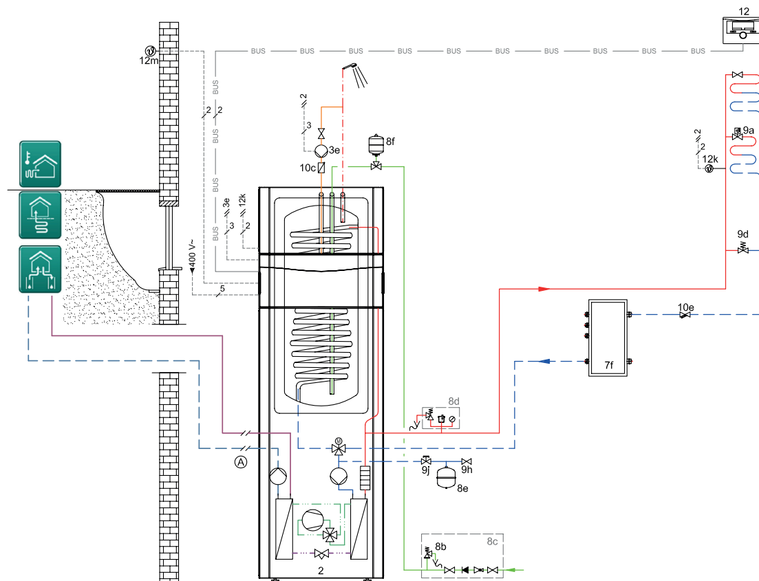
Installatievoorbeeld 2: flexoCOMPACT VWF ..8/4 met 2 verwarmingscircuits en een buffervat als hydraulische scheiding
