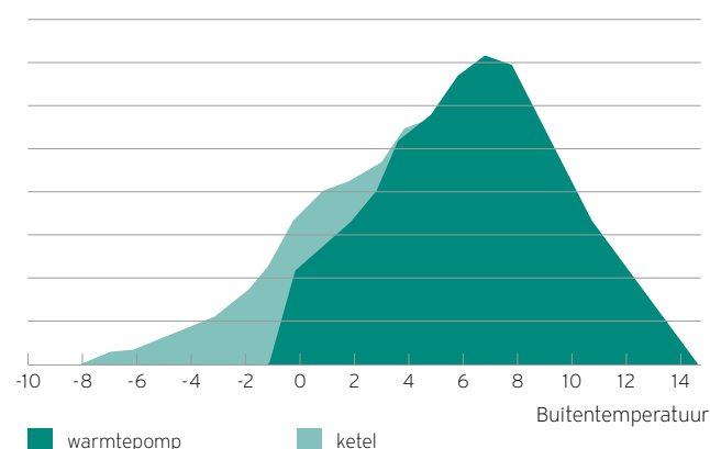
Warmtevraag door warmtepomp en ketel
