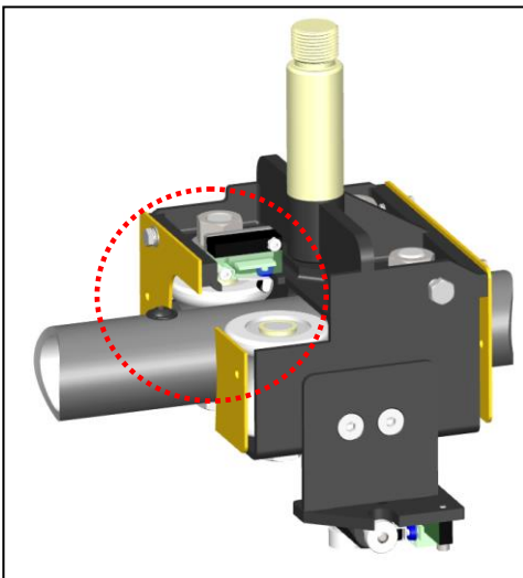
Position des Notendschalters am unteren Rollensatz
