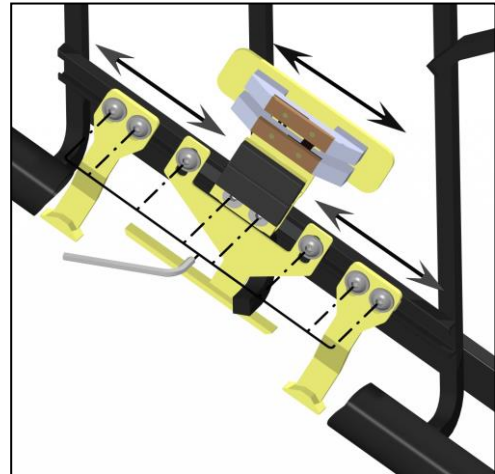
Umgehungsschalter-, Riegelkurven und Ladestation (mittlere Haltestelle)
