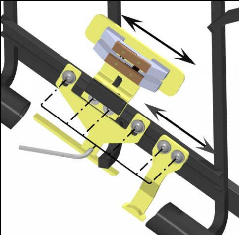
Umgehungsschalter-, Riegelkurven und Ladestation (obere Haltestelle)
