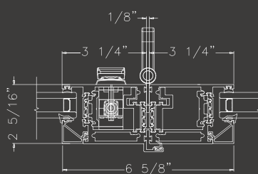
Hinge Stile Dropbolt 2P - Flat Hinge
