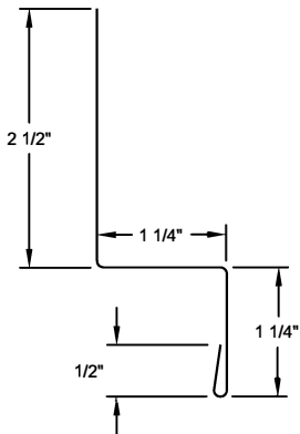
Double Angle DA-2
