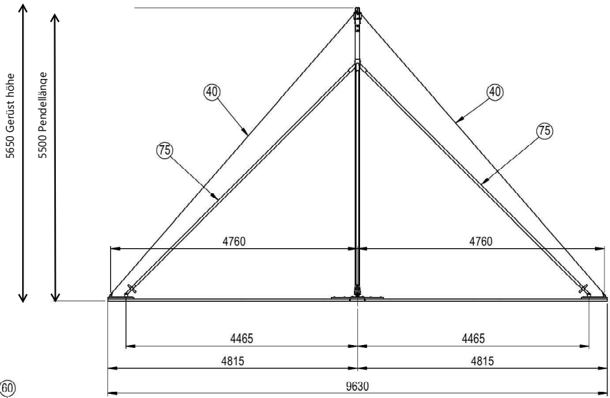
Ansicht D (M1:50)
