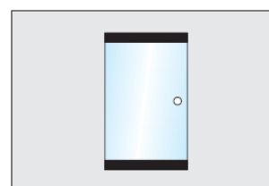
top door rail bottom door rail max. 1.400 x 2.800 mm max. 140 kg
