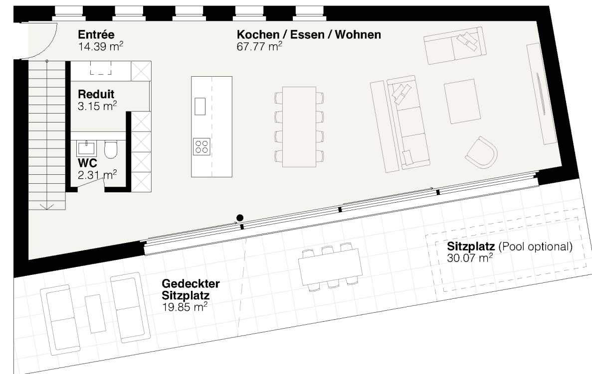
Erdgeschoss
