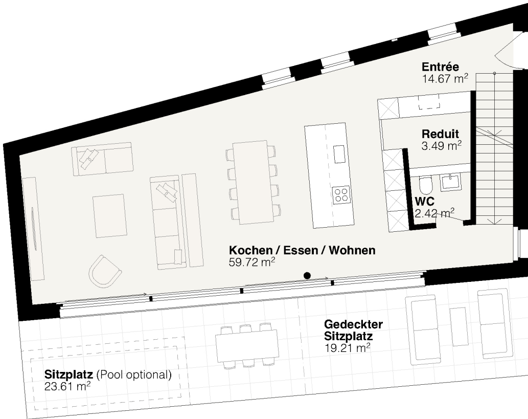
Erdgeschoss
