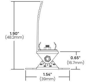
Pivot Metal Glare Shield
