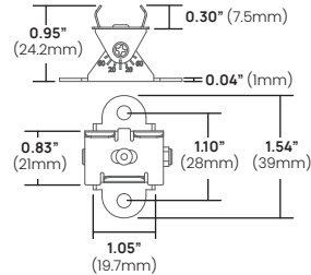
Metal Pivot Clip
