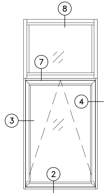
P.O./FIXED WINDOW
