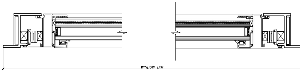
FLANGE FRAME
