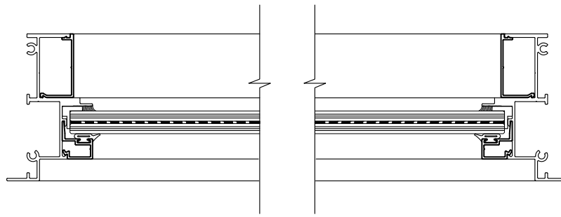
FLANGE FRAME
