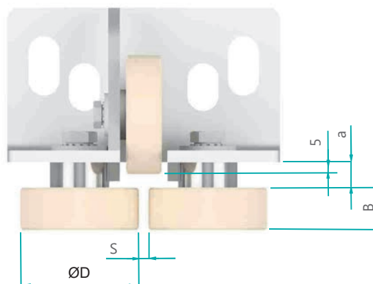
GUIDAGE À GALETS: RFL
