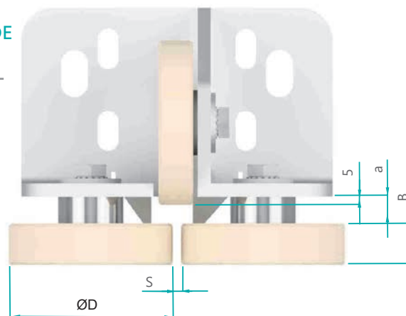
GUIDAGE À GALETS: RFS
