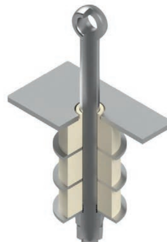
VERSION 3 - type A + type B + type B COURBE VERTE
