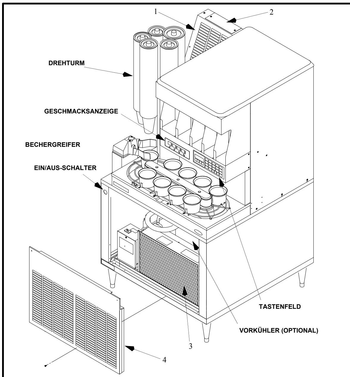
Automatisiertes Getränkesystem — Abbildung des vollständigen Geräts
