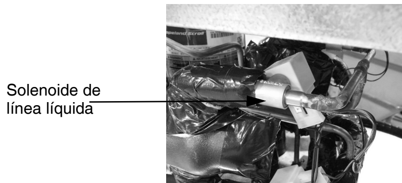
Figura 51. Solenoide Línea Líquido (1 Barril)
