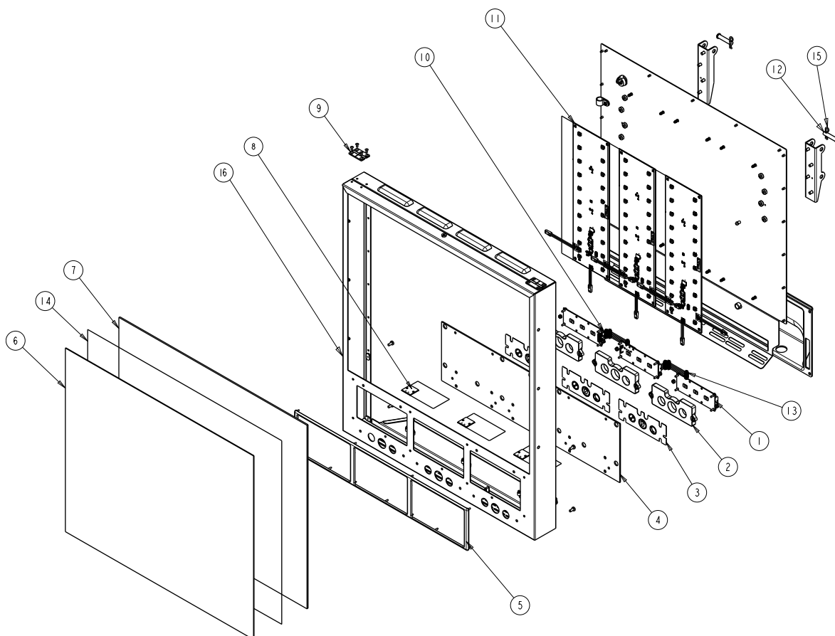
Figure 8. Assemblée Présentoir Assembly (Grand)
