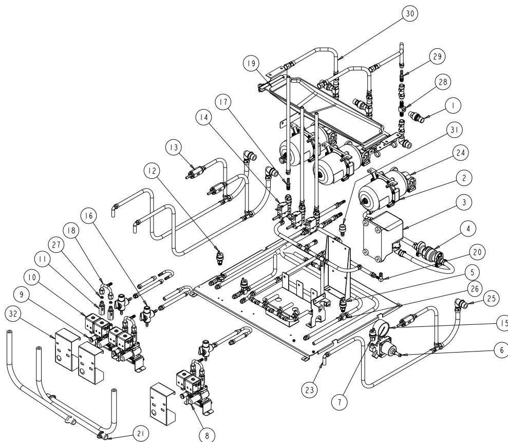
Figure 5. Système de Livraison Produit
