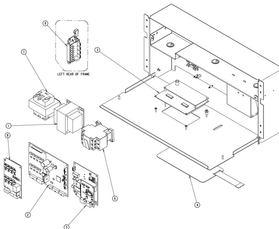
Figure 7. Boîte d'Assemblé Électronique
