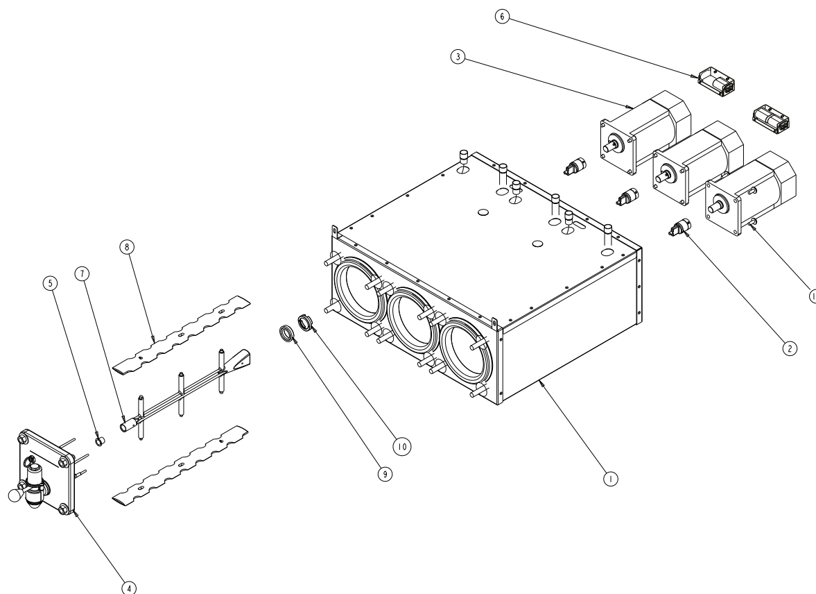
Figure 2. Emballage Mousse/ Assemblé Moteur
