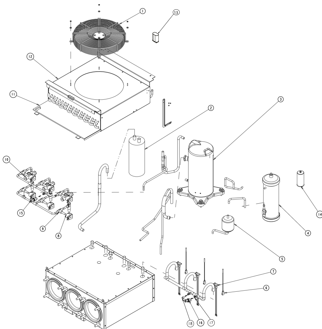
Figure 6. Système de Réfrigération
