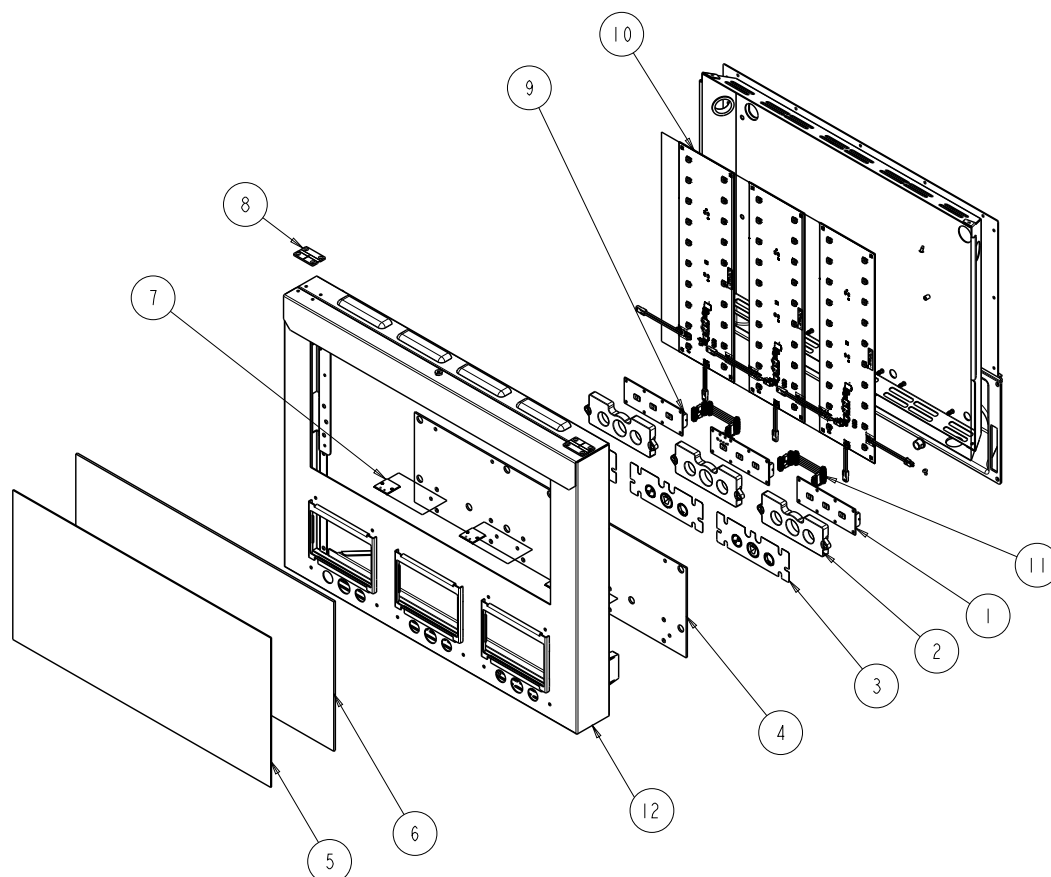
Figure 9. Assemblage présentoir (Modifié Court)
