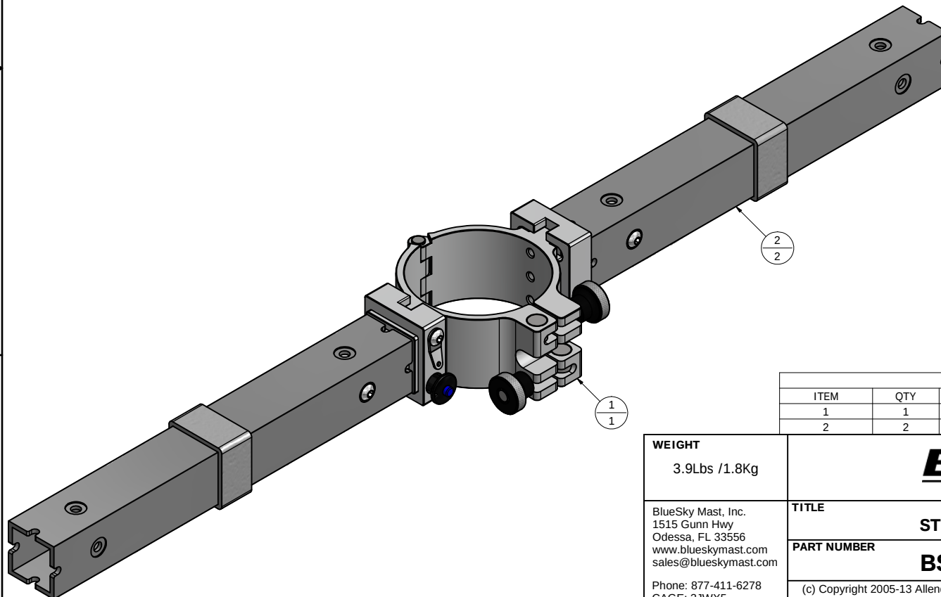
BSM3-P-A352-T00-000 POLE MOUNT-AL3-TWO WAY
