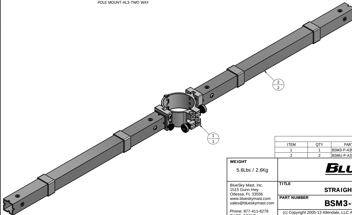
BSM3-P-A352-T00-000 POLE MOUNT-AL3-TWO WAY
