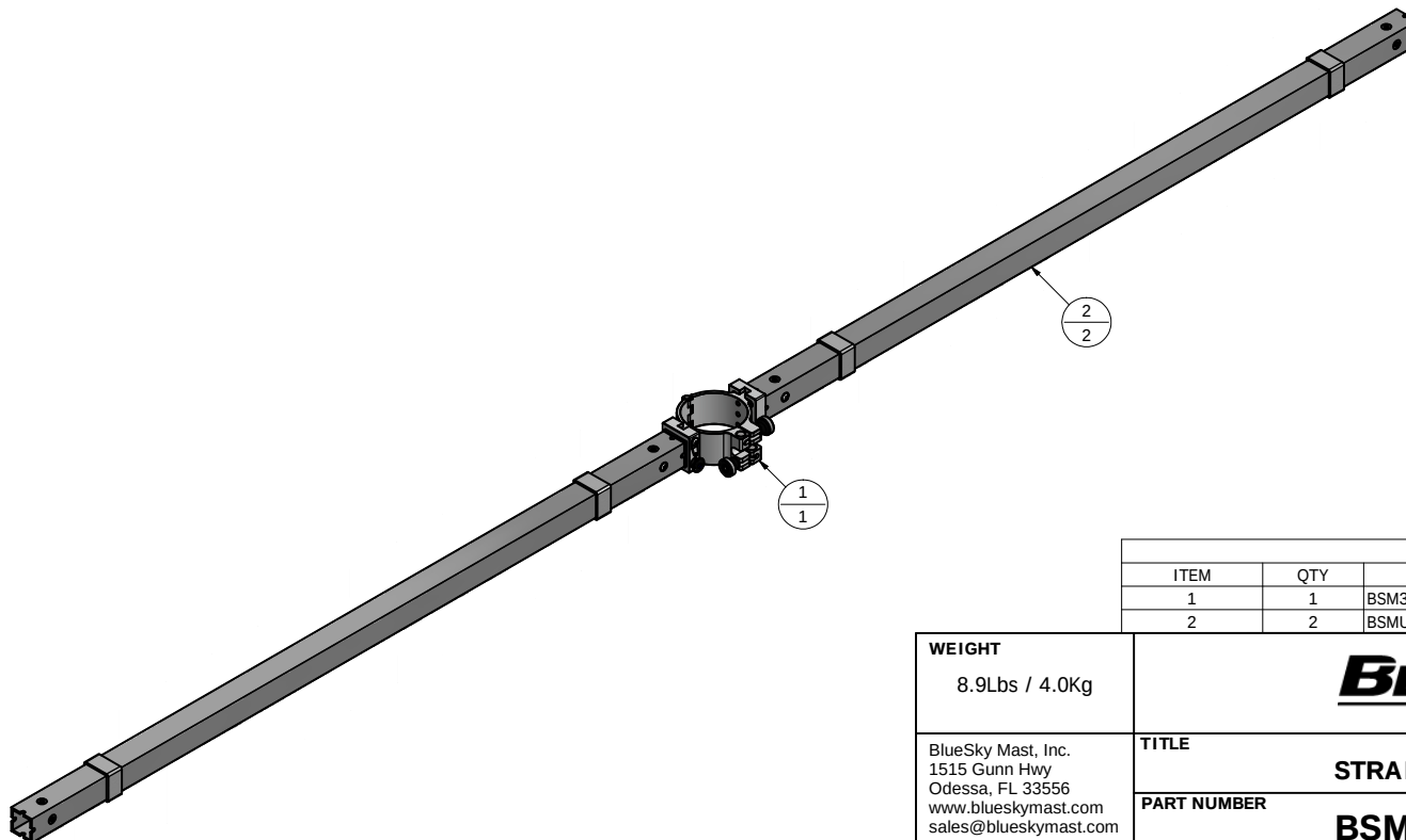
BSM3-P-A352-T00-000 POLE MOUNT-AL3-TWO WAY
