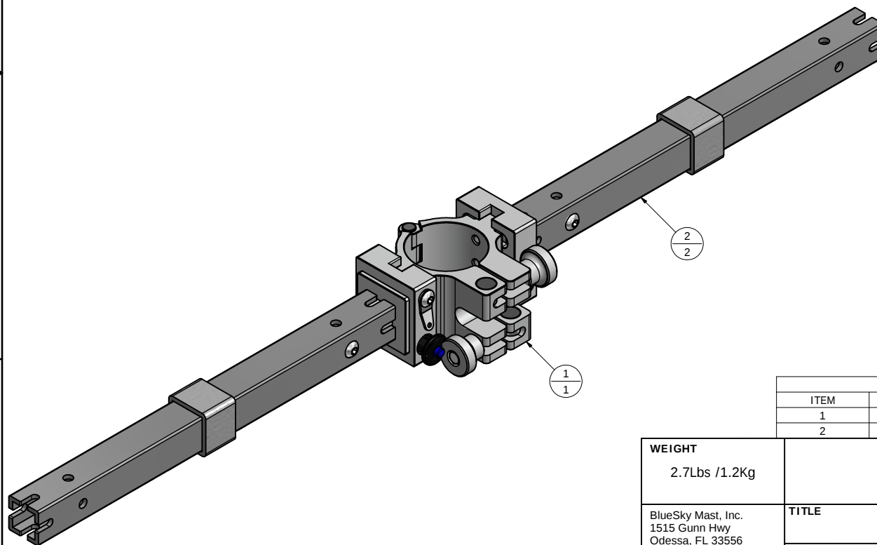
BSM2-P-A352-T00-000 POLE MOUNT-AL1/AL2-TWO WAY
